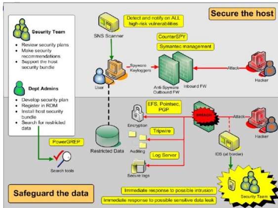
Gambar Penempatan Konfigurasi Tripwire
