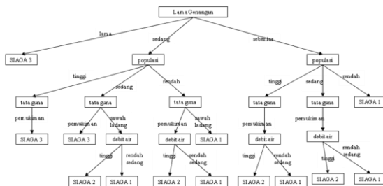
Gambar 6. Contoh Tree yang digunakan dalam program
