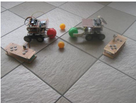
Gambar 3.1 Integrasi robot soccer dengan remot control
