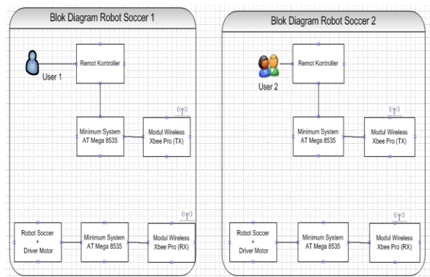
Gambar 2.1 Blok Diagram Sistem
