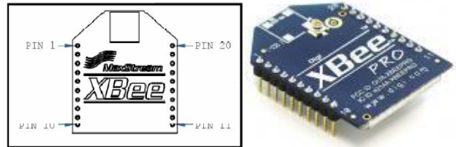
Gambar 2.6 Bentuk & Pin Xbee Pro
