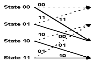
Gambar 5 hubungan input,output,state dan next state pada encoder kode konvolusi
