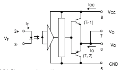
Gambar 2.3. rangkaian opto TLP 250
