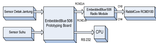
Gambar 3.1 Blok Diagram Perangkat Keras
