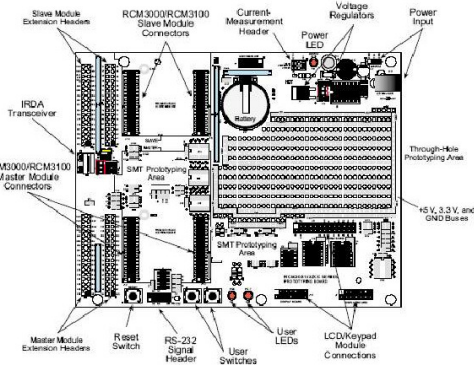
Gambar 2.2 Bentuk Fisik Prototyping Board
