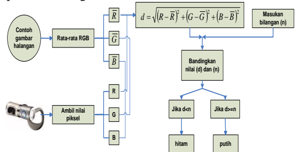
Gambar 6. Blok diagram segmentasi Halangan
