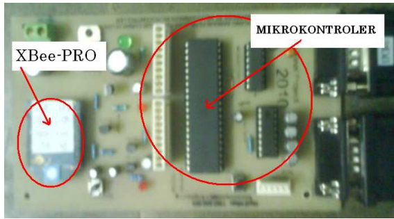
Gambar 4. Rangkaian Pemancar
