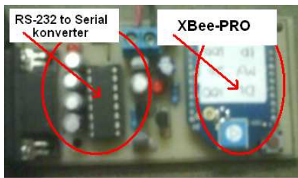
Gambar 5. Rangkaian Penerima
