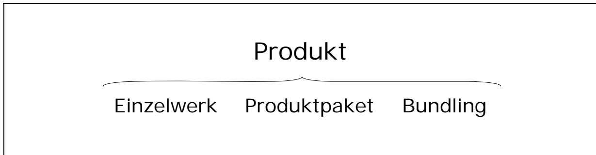
Abbildung 3.1/1: Produktverständnis
