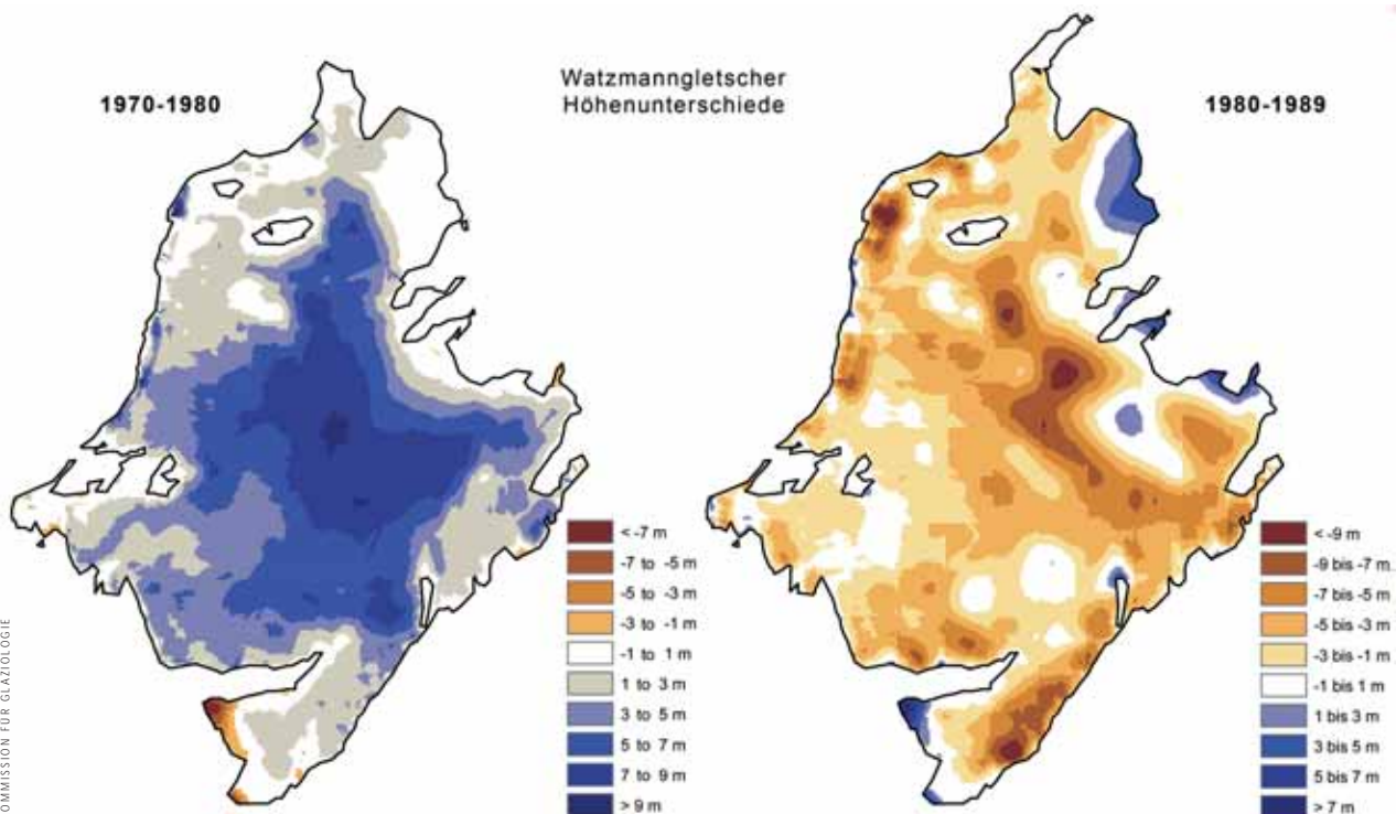
Abb. 4: Höhenänderungen (in Metern) am Watzmanngletscher von 1970 bis 1980 und von 1980 bis 1989.
