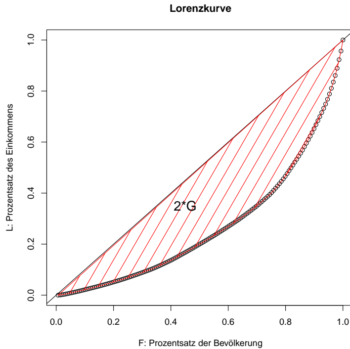
Abbildung 2.1: Die Lorenzkurve
