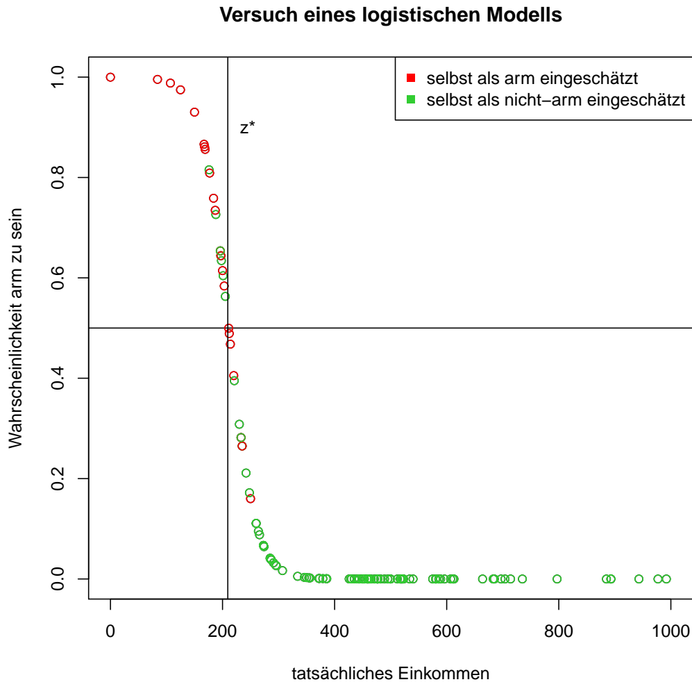
Abbildung 4.6: Logistische Regression
