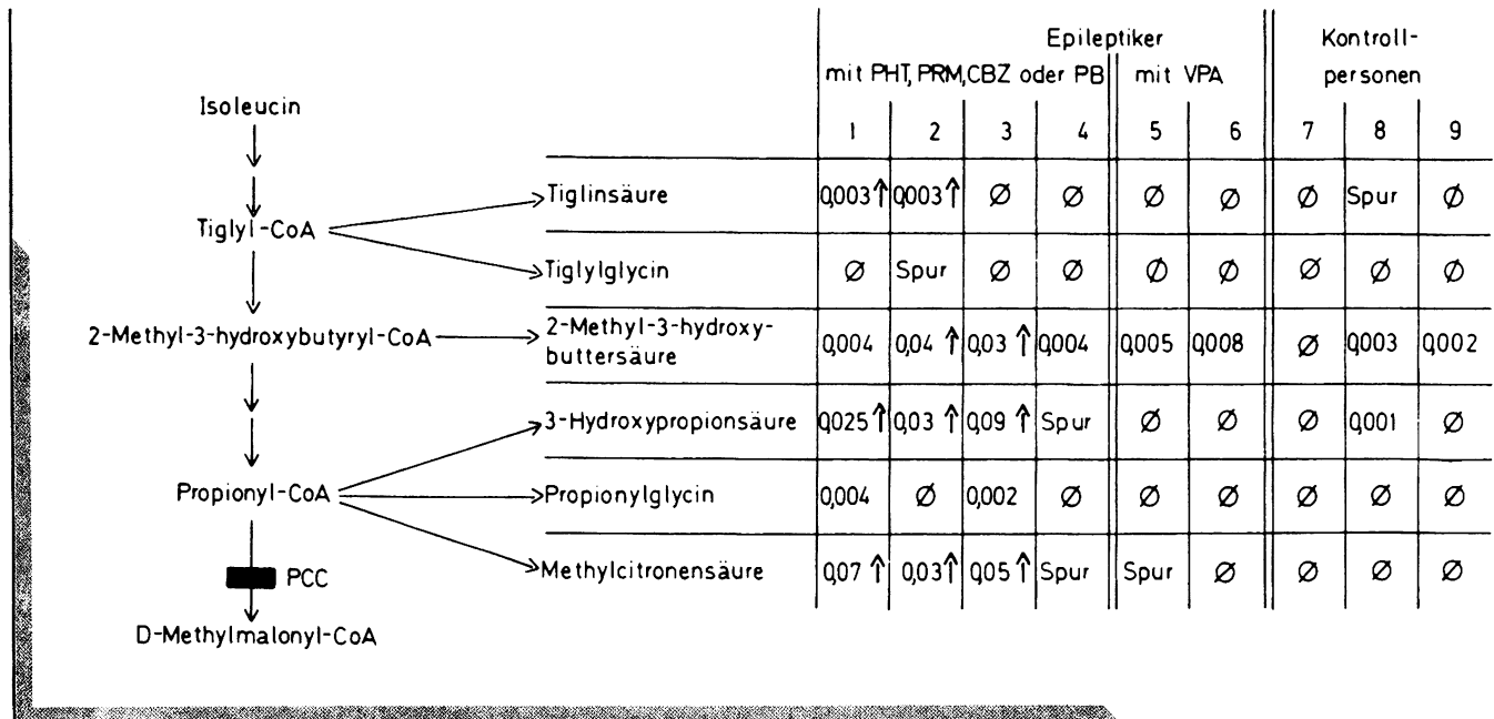
Abbildung 1 Beim Abbau von Isoleucin auftretende Säuren im Urin ( \mu\text{mol}/\text{mg} Kreatinin) bei 6 Epileptikern (PHT = Phenytoin, PRM = Primidon, CBZ = Carbamazepin, PB = Phenobarbital, VPA = Valproat) und drei Kontrollpersonen; PCC = Propionyl-CoA-Carboxylase, ↑ = erhöht
