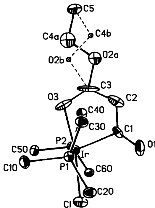
Abb. 1. Struktur von 1 im Kristall. Ausgewählte Bindungsabstände (pm) und Bindungswinkel (°): Ir–C1 203.4(11), Ir–O3 206.9(8), Ir–Cl 233.8(3), Ir–P1 233.4(3), Ir–P2 234.0(3), C1–C2 136.8(20), C1–O1 117.8(14), C2–C3 133.9(27), C3–O3 129.8(24), P1–Ir–P2 169.3(1), C1–Ir–O3 171.4(3), C1–Ir–C1 107.4(3), C1–Ir–O3 81.3(4), Cl–Ir–P1 89.8(1), O3–Ir–P1 89.9(2), C1–Ir–P1 94.6(3), C1–Ir–P2 96.0(3), C1–Ir–O3 81.3(4), O3–Ir–P2 89.9(2), Ir–C1–C2 109.4(9), C1–C2–C3 118.2(14), C2–C3–O3 121.8(12), Ir–O3–C3 109.0(9).
