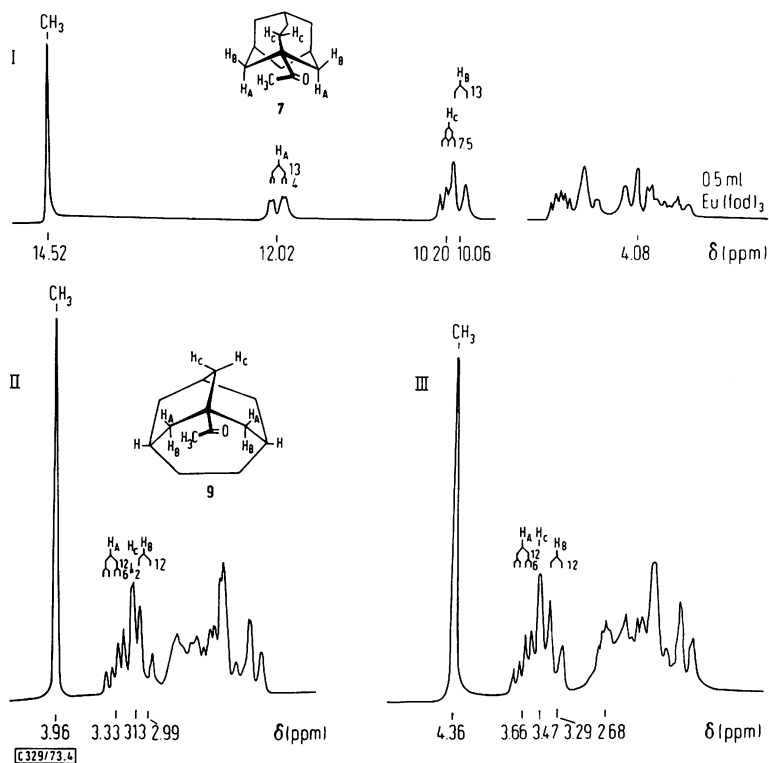
Abb. 4. ^1\text{H} -NMR-Spektren des 3-Homoadamantylmethylketons (7) (I) und des 1-Homoadamantylmethylketons (9) (II, III) in \text{CCl}_4 (100 MHz) unter Zusatz von \text{Eu}(\text{fod})_3 (I) bzw. \text{Eu}(\text{DPM})_3 (II, kleine Konz.; III, höhere Konz.)
