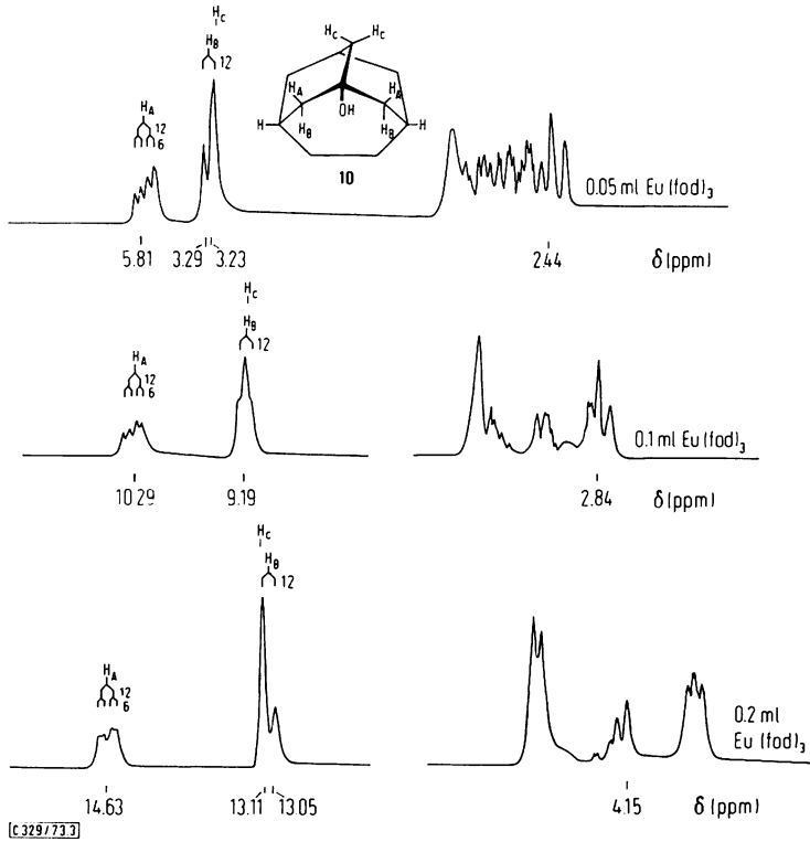
Abb. 3. 1 H-NMR-Spektren des Homoadamantan-1-ols ( 10 ) in CCl 4 unter Zusatz von Eu(fod) 3 -Lösung (s. Exp. Teil)
