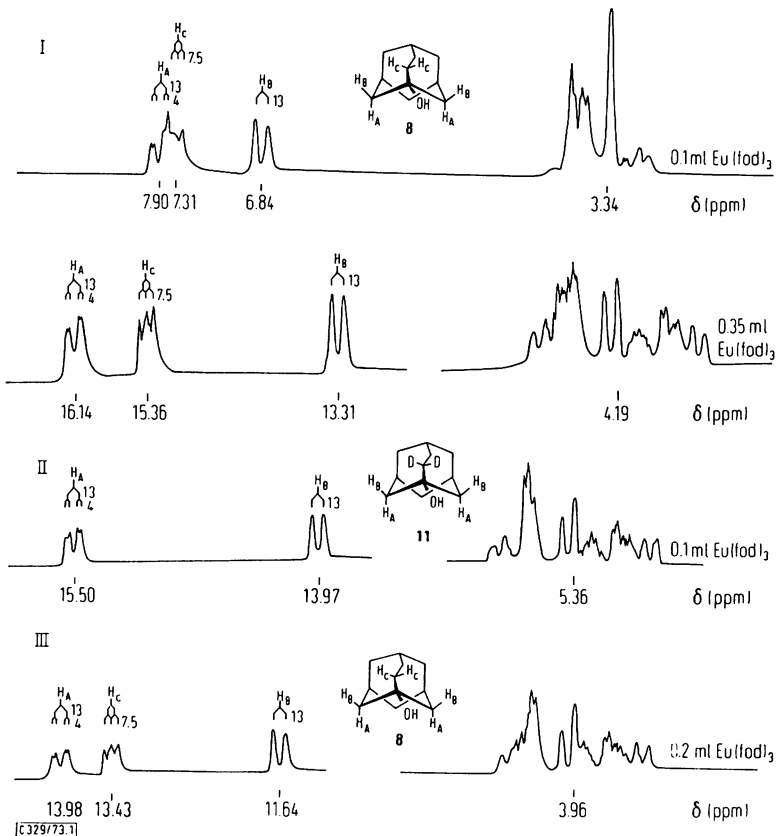
Abb. 1. ^1\text{H-NMR} -Spektren des Homoadamantan-3-ols ( 8 ) in \text{CCl}_4 (100 MHz) unter Zusatz von \text{Eu}(\text{fod})_3 (s. Exp. Teil)
