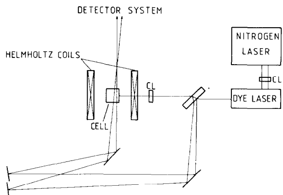
Fig.2. Apparatus.
