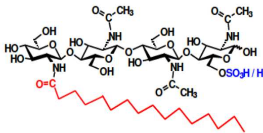
D Hexamère de CO
