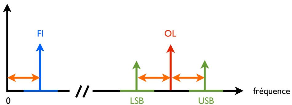
FIGURE 1.16 – Principe de la technique hétérodyne au niveau fréquentiel.
