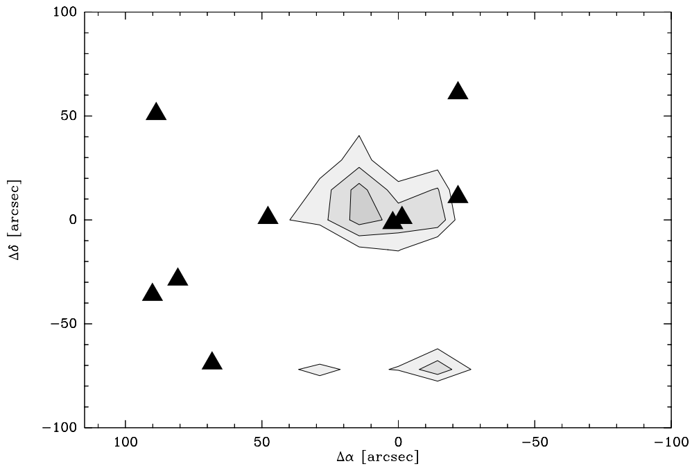
FIGURE A.16 – Carte intégrée en vitesse de la transition de \text{CH}_3\text{CCH} à 85.457\text{ GHz} obtenue avec le télescope de l'IRAM. Les contours représentent 0.3, 0.4\text{ et }0.5\text{ K.km s}^{-1} . Le rms est de 0.18\text{ K} .
