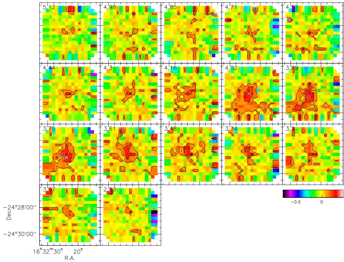
FIGURE A.8 – Carte de la transition de CH 3 CCH à 85.457 GHz en fonction des canaux de vitesse obtenue avec le télescope de l'IRAM.
