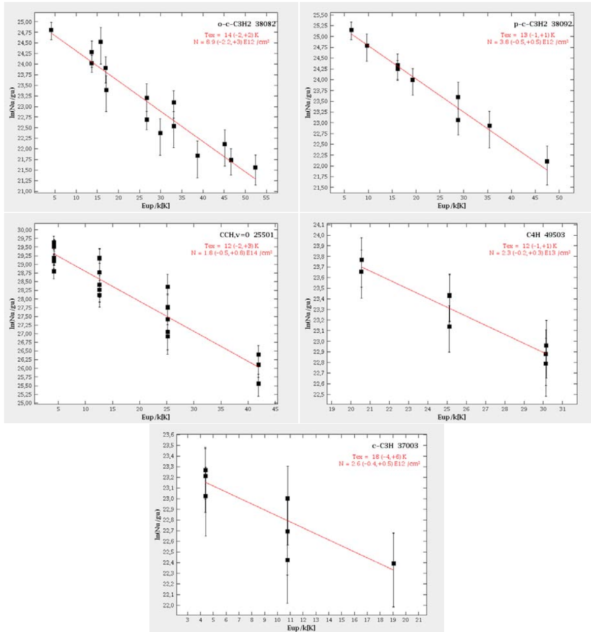
FIGURE A.1 – Diagrammes rotationnels des espèces ortho- c-C_3H_2 , para- c-C_3H_2 , CCH, C_4H et c-C_3H détectées dans le relevé spectral TIMASSS sans correction de dilution.
