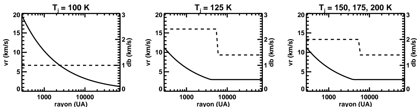
FIGURE 5.5 – Représentation en fonction du rayon des profils de vitesse d’effondrement (en trait plein) et du paramètre b -doppler (en pointillés) utilisés pour modéliser les raies de HDO dans la source G34 avec différentes températures de saut en abondance T_j = 100, 125, 150, 175 et 200 K.
