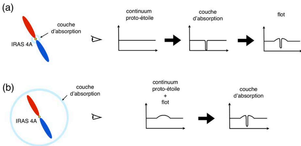
FIGURE 4.5 – Représentation des différentes positions possibles de la couche d’absorption par rapport à la source IRAS 4A et son flot moléculaire et impact sur l’absorption des raies fondamentales. Dans le cas (a), la couche d’absorption est peu étendue par rapport aux flots. Le continuum qui va être absorbé est uniquement dû à la proto-étoile. La composante large produite par les flots s’ajoute dessus. Dans le cas (b), la couche d’absorption est plus étendue que les flots moléculaires. Le continuum qui va être absorbé est donc dû à la proto-étoile et au flot moléculaire.
