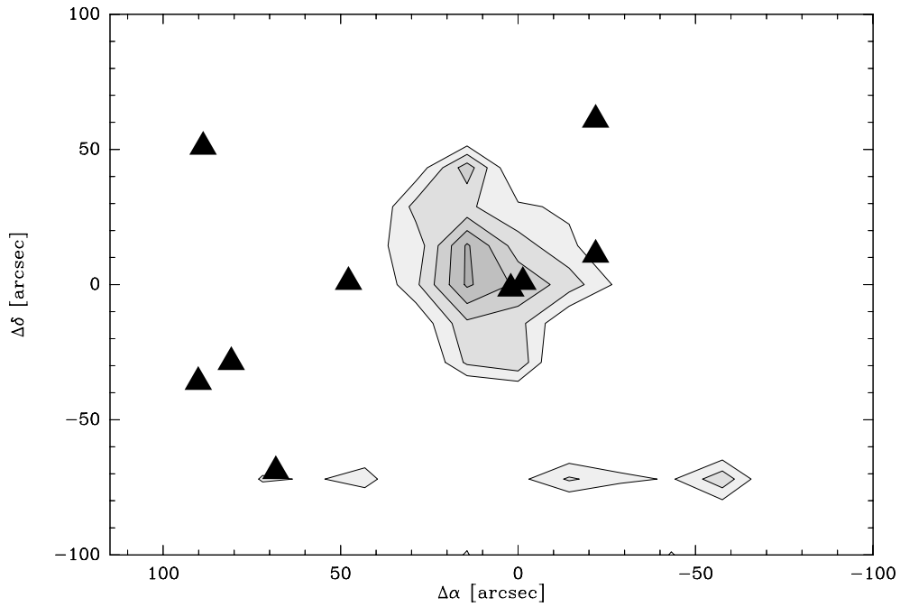
FIGURE A.15 – Carte intégrée en vitesse de la transition de \text{CH}_3\text{CCH} à 85.456\text{ GHz} obtenue avec le télescope de l'IRAM. Les contours représentent 0.2, 0.25, \dots 0.4\text{ K.km s}^{-1} . Le rms est de 0.18\text{ K} .
