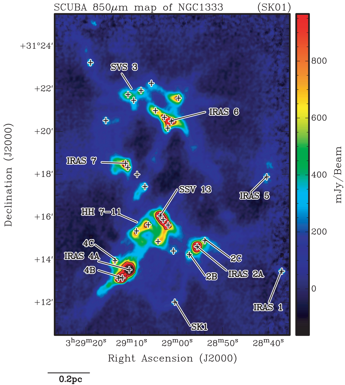
FIGURE 4.1 – Carte du continuum de la poussière à 850 \mu m dans NGC 1333 (Sandell & Knee 2001). Les contours représentent 10%, 20%, 30%, ..., 90% du flux maximum de 6.68 Jy beam -1 . Les symboles + indiquent les positions des sources de continuum SCUBA identifiées par Sandell & Knee (2001).
