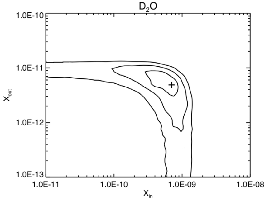
FIGURE 3.22 – Contours de \chi^2 à 1σ, 2σ et 3σ obtenus en ajoutant à la structure une couche d'absorption avec N(\text{para-D}_2\text{O}) = 1.1 \times 10^{12} \text{ cm}^{-2} et N(\text{ortho-D}_2\text{O}) = 1.4 \times 10^{12} \text{ cm}^{-2} . Le meilleur modèle est représenté par le symbole “+” et a été obtenu avec la méthode de \chi^2 n° 2.
