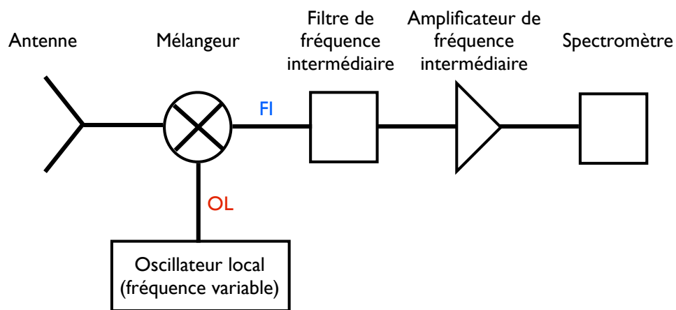
FIGURE 1.15 – Schéma d'un récepteur hétérodyne.
