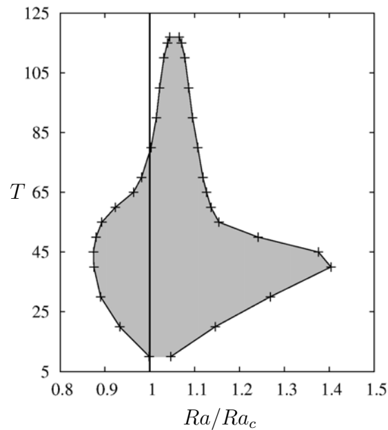
FIGURE 6.13 – Région d'existence des convectons dans le plan (Ra, T) . Le trait plein vertical représente le seuil d'instabilité amenant la convection stationnaire. La région d'existence est délimitée par le premier et le dernier noeud-col de la branche de convectons. Dans les cas où il n'y a pas de noeud-col, le point de bifurcation fait office de délimiteur.
