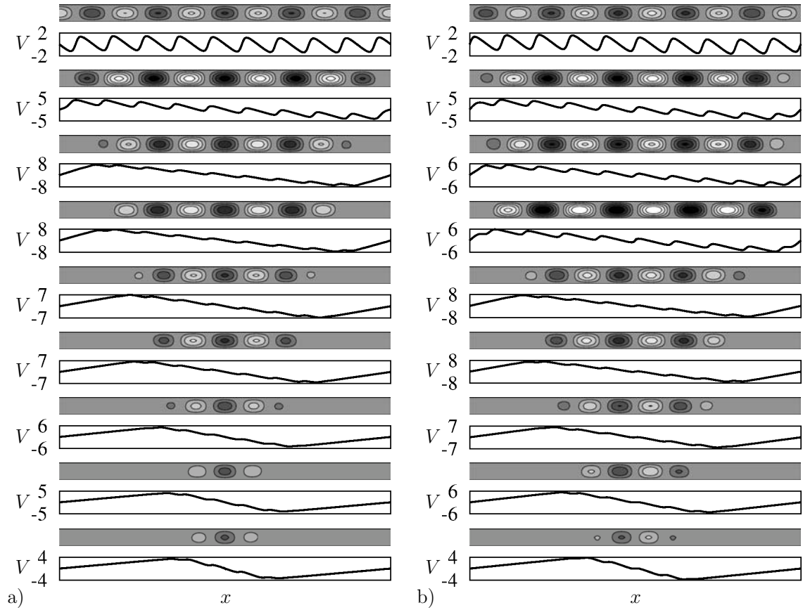
FIGURE 6.6 – Solutions aux noeuds-cols successifs des branches (a) L_{10}^- , (b) L_{10}^+ de la figure 6.5. Les tracés supérieurs montrent les isovaleurs de la fonction de courant. Les tracés inférieurs montrent le profil de V(x) \equiv \int_0^1 v(x, z) dz . Les solutions du haut ont été prises au voisinage du point de reconnection sur P_5 .
