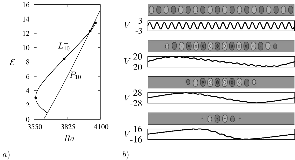
FIGURE 6.14 – (a) Diagramme de bifurcation pour la branche de convectons pairs L_{10}^+ à T = 70 , \sigma = 0.6 et \Gamma = 10\lambda_c (voir figure 6.12). La branche L_{10}^+ bifurque et termine sur la même branche : P_{10} . Les points représentent les solutions tracées en (b). La même représentation que pour la figure 6.11 a été utilisée.
