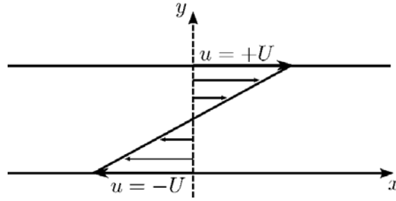
FIGURE 2.20 – Représentation schématique de l’écoulement de Couette. L’écoulement est généré par le mouvement en sens opposé des parois confinant le fluide dans la direction y . Cette configuration entraîne la présence d’un état laminaire dont la vitesse est linéaire avec y .
