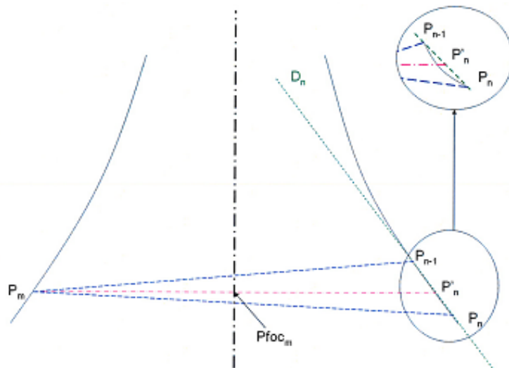
FIGURE 4.5 – Principe de l'algorithme de l'autofocus.
