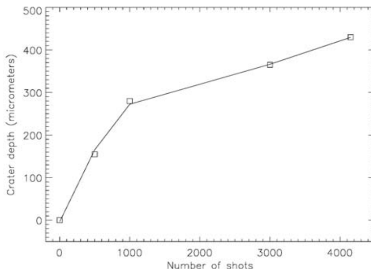
FIGURE 6.5 – Dépendance de la profondeur du cratère selon le nombre de tirs (corrélation d'ordre 3).
