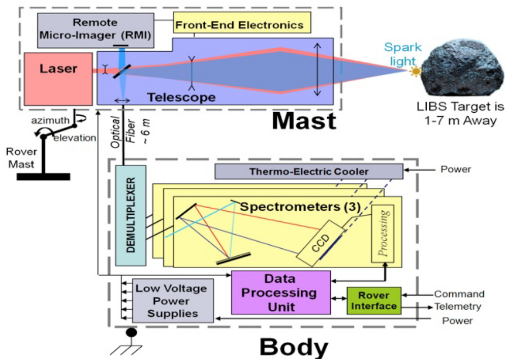
FIGURE 3.1 – Schéma de ChemCam.
