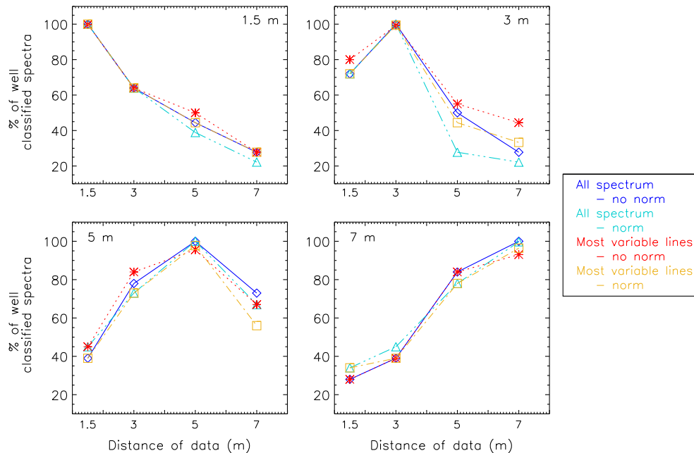
FIGURE 7.9 – Comparaison des résultats obtenus pour chacun des modèles utilisés, selon les paramètres pris en compte. Chaque graphique représente un modèle utilisant une distance pour classer les données de chacune des distances. La distance du modèle est indiquée sur chaque graphique.
