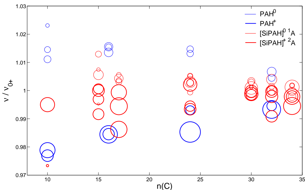
Fig. 3.8: Rapport des fréquences \nu_{CC} les plus élevées pour les PAH 0/+ et les complexes \pi [SiPAH] 0/+ sur les fréquences moyennes correspondantes des PAH 0/+ \nu_{0+} = \frac{\nu_0 + \nu_+}{2} .
