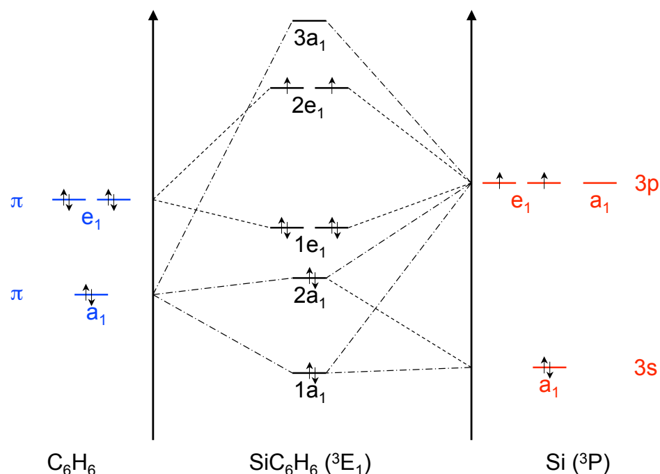
Fig. 3.6: Diagramme d'orbitales moléculaires du système \pi [SiC 6 H 6 ] triplet dans le groupe de symétrie C_{6v} . Traits pointillés continus : interactions à deux orbitales de type e_1 ; traits pointillés discontinus : interactions à trois orbitales de type a_1 .
