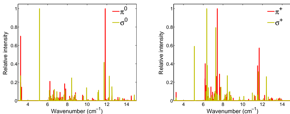
Fig. 7.7: Spectres harmoniques calibrés des complexes formés avec la molécule C_{24}H_{12} \sigma^0 et \pi^0 (gauche), \sigma^+ et \pi^+ (droite) calculés au niveau B3LYP/D95++**.
