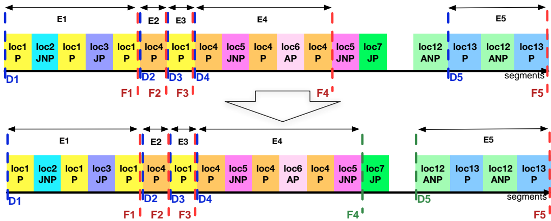
FIGURE 4.10 – Macro-segmentation fondée sur les rôles : affinement des frontières de chaque zone E_j .
