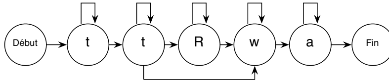
FIGURE 5.1 – Structure simplifiée du Modèle de Markov associé à la prononciation du mot "trois"
