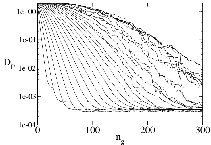
FIGURE 4.4.: Distance D_P(n_g) entre la distribution P(l) et \tilde{P}(l) en fonction du nombre de portes n_g pour n_q = 2, 3, \dots, 28 qubits (de gauche à droite).
