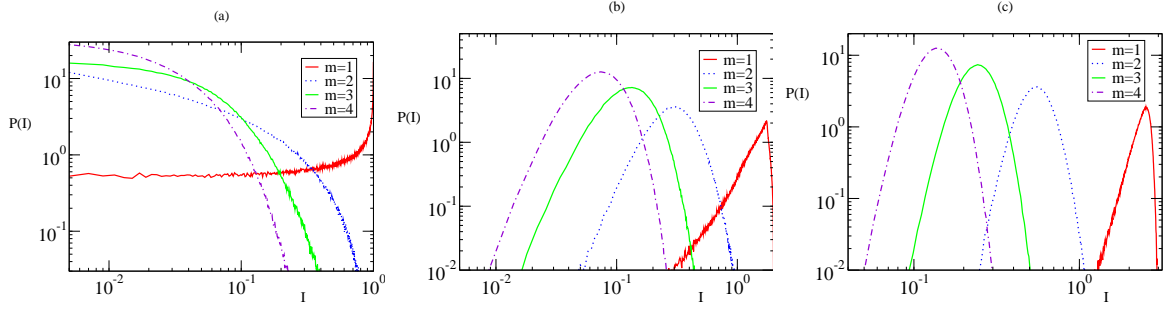
FIGURE 3.1.: Distributions de l'interférence représentés en échelle log-log, calculées numériquement à x = 0.1 pour n = 2, 3, 4 (graphes (a), (b) et (c) respectivement). Dans chaque graphe m varie entre 1 et 4. Dans chaque cas le nombre de réalisations statistiques vaut n_r = 10^6 .
