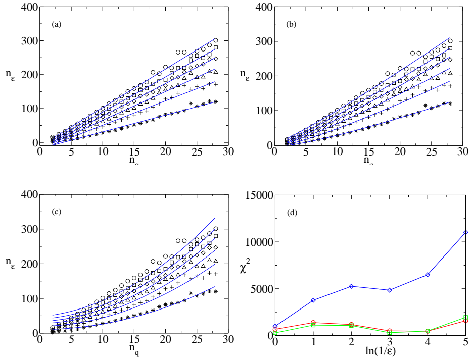
FIGURE 4.5.: Nombre de portes n_\epsilon nécessaire pour atteindre D_p \leq \epsilon pour \ln(\epsilon) = 0, -1, -2, -3, -4 et -5 ( * , + , \Delta , \diamond , \square , \circ respectivement) et n_q = 2 \dots 28 . Les lignes droites représentent les modèles de fonctions f_1 , f_2 et f_3 (1 ier , 2 ième et 3 ième graphique respectivement). Le dernier graphique représente le \chi^2 pour ces modèles ( f_1 ( \circ ), f_2 ( \square )), et f_3 ( \diamond ).
