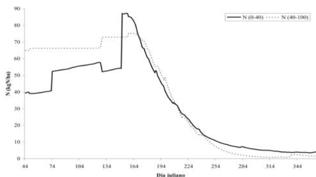
Fig. 3. Evolución diaria de la cantidad de nitrógeno presente en el suelo (kg N/ha) de 0 a 40 cm y de 40 a 100 cm para Habitual.
