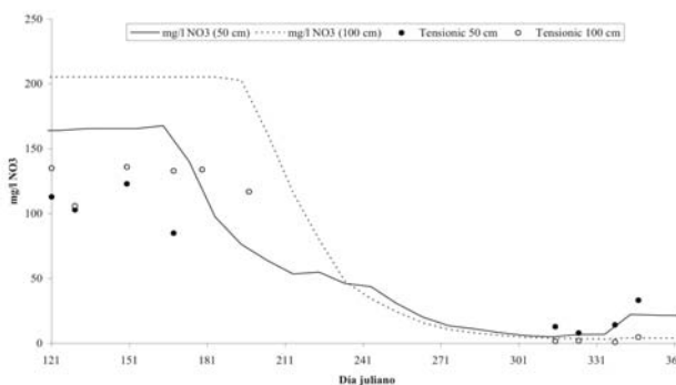
Fig. 2. Evolución de la concentración en nitratos (mg/l NO 3 ) en las aguas del suelo según modelo y según analítica para Habitual.
