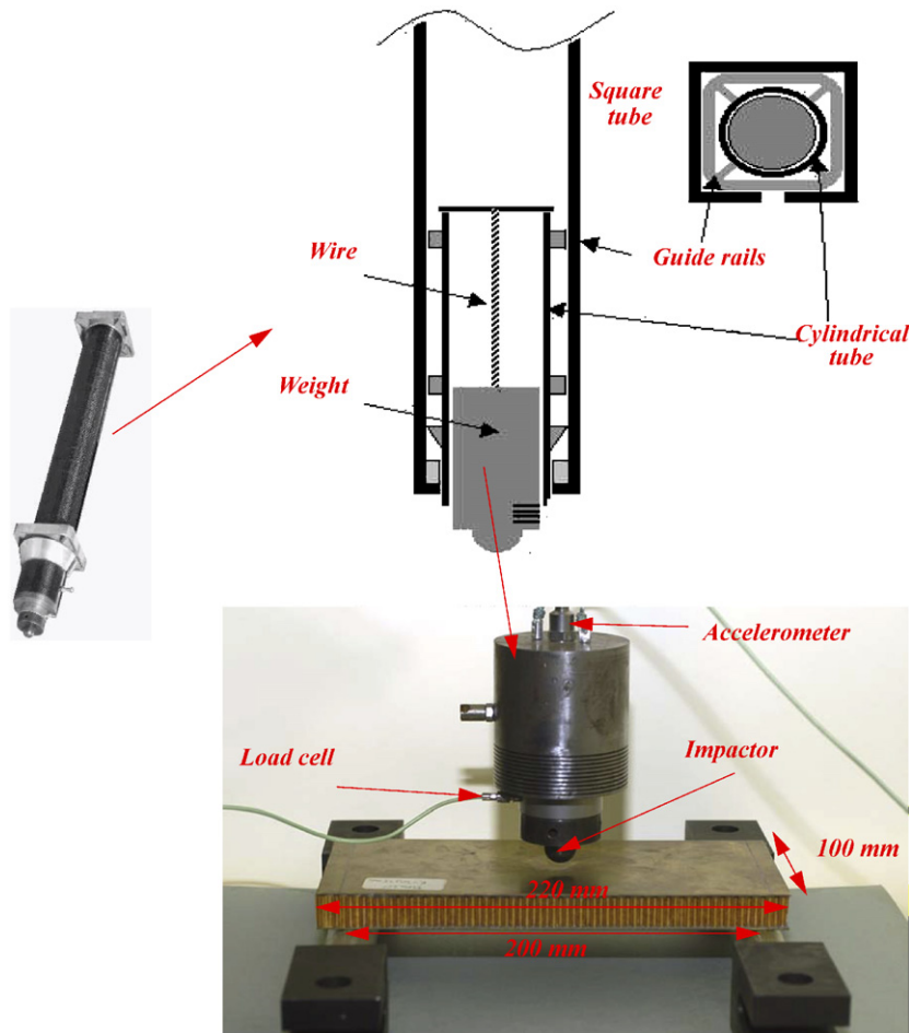
Fig. 19. Load drop test rig.
