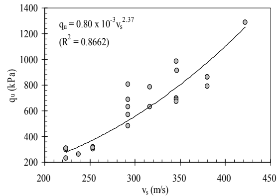
Fig. 9: q_u - v_s
