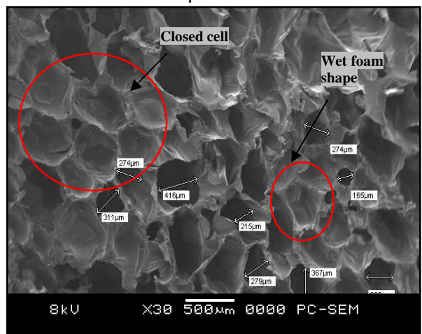
Fig. 6. PU cell surface
