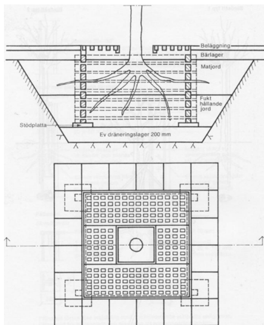
Figur 15. Trädgrop i hårdjord yta enligt Mark AMA 72 (Mark AMA 72).
