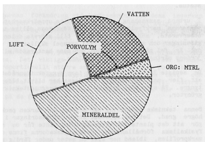
Figur 14. Schematisk framställning av markens huvudkomponenter (Rolf, 1986).
