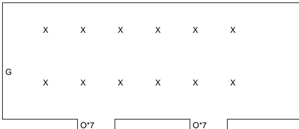
Figur 3: Översiktsbild i stall II. X= tilluftsfläktar. O= 7 frånluftsfäläktarna. Dessa är placerade i två fläktrum som man ser på bilden ovan. I fläktrummet så är de placerade i vägen i två rader, en undre rad med tre stycken fläktar i och en övre rad med fyra stycken fläktar i. G= Gavelfläkt (stor fläkten)
