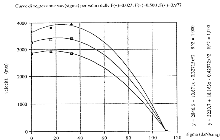
Fig. 7 Curve di possibilità tensionale per sforzo di compressione semplice
