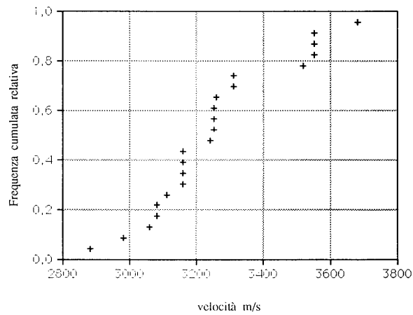
Fig. 2 Diagramma di distribuzione cumulativo della velocità Vp condizionato dal valore \sigma = 0
