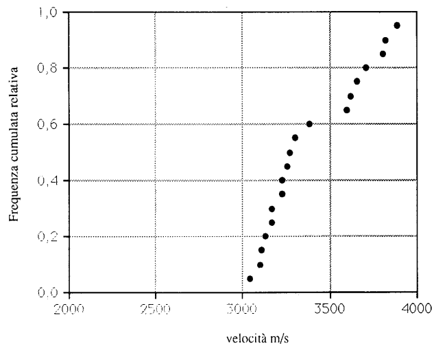
Fig. 4 Diagramma di distribuzione cumulativo della velocita Vp condizionato dal valore \sigma = 1000 KN
