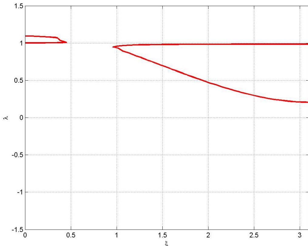
Figura 5.18 – Andamento degli autovalori del modello pseudo-continuo non ritardato.
