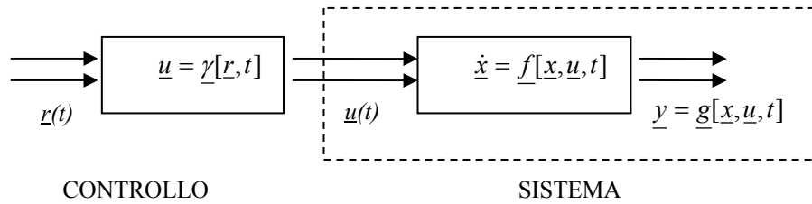
Figura 5.2 – Processo di modellizzazione dello spazio di stato con funzione di controllo.
