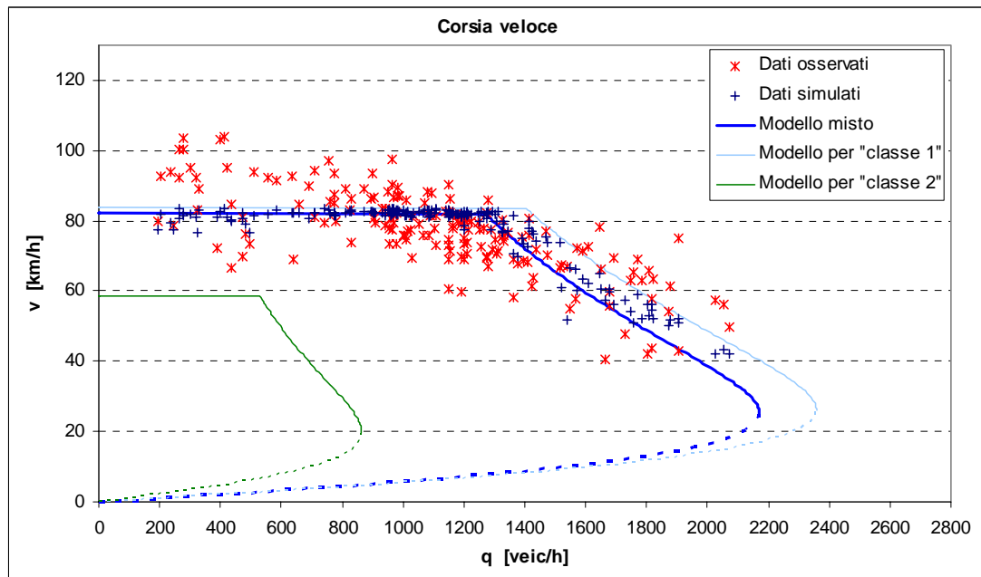
Figura 4.5 – Risultati della calibrazione con sedici parametri – corsia veloce.
