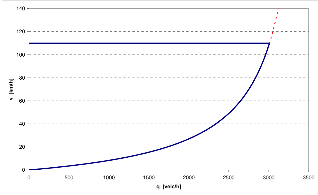
Figura 3.6 – Relazione velocità e flusso per b = \hat{b} .
