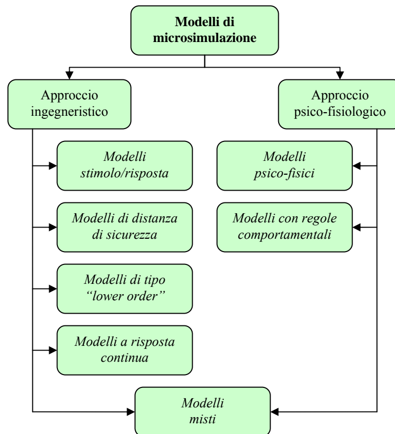
Figura 1.1 – Approcci dei modelli microscopici di moto longitudinale
