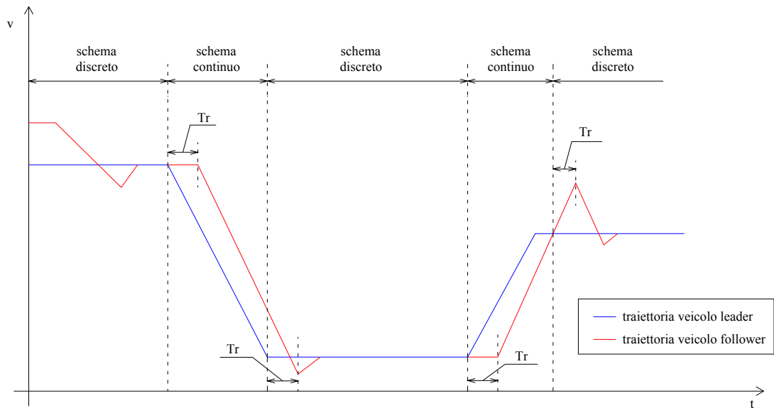
Figura 5.27 – Possibile andamento dei veicoli secondo il modello predittivo misto.
