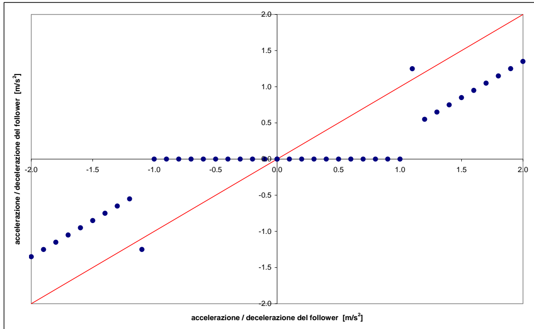
Figura 2.8 – Confronto tra le accelerazioni di leader e follower (modello di Newell).
