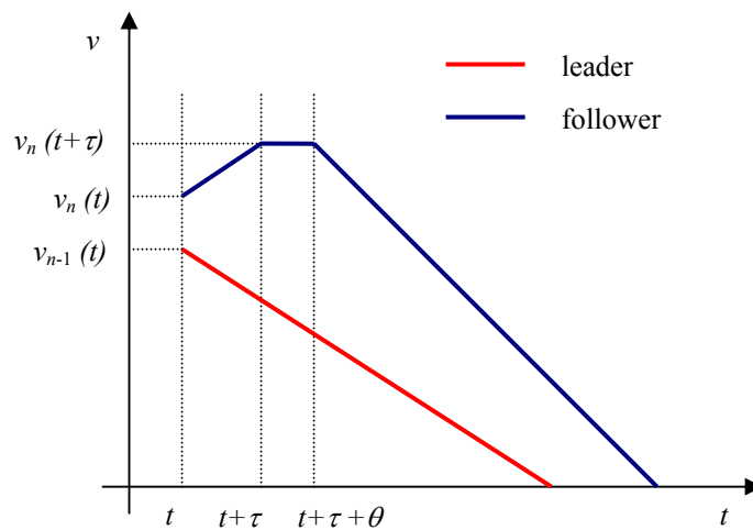
Figura 3.2 – Profilo di velocità per il calcolo della velocità di Gipps.
