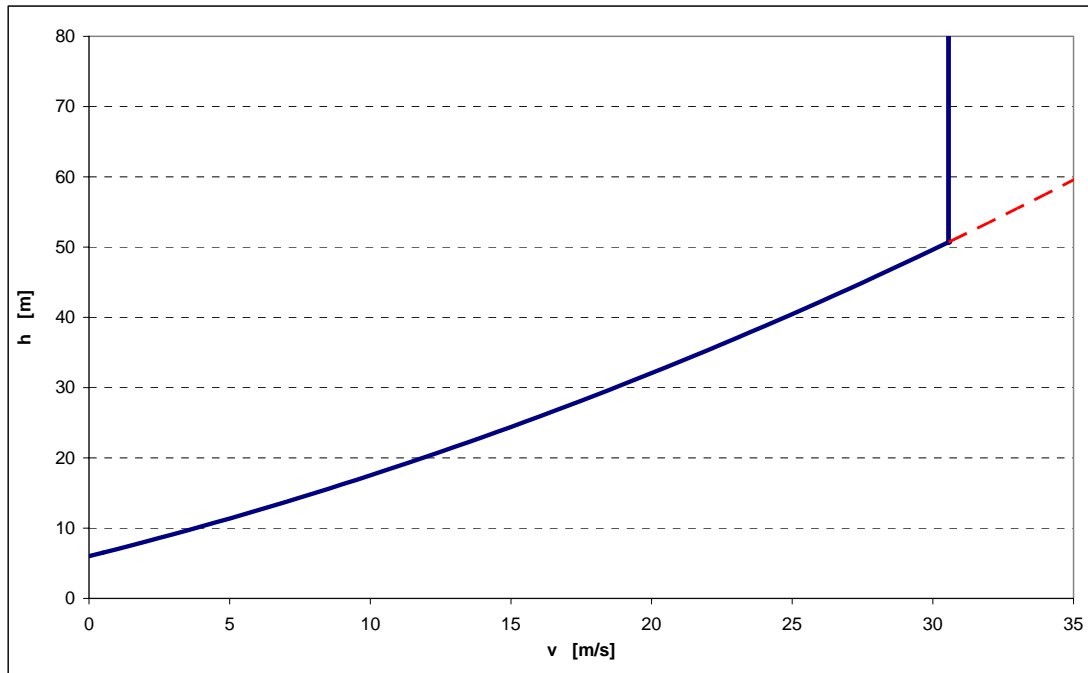
Figura 3.7 – Relazione distanziamento e velocità per b < \hat{b} .
