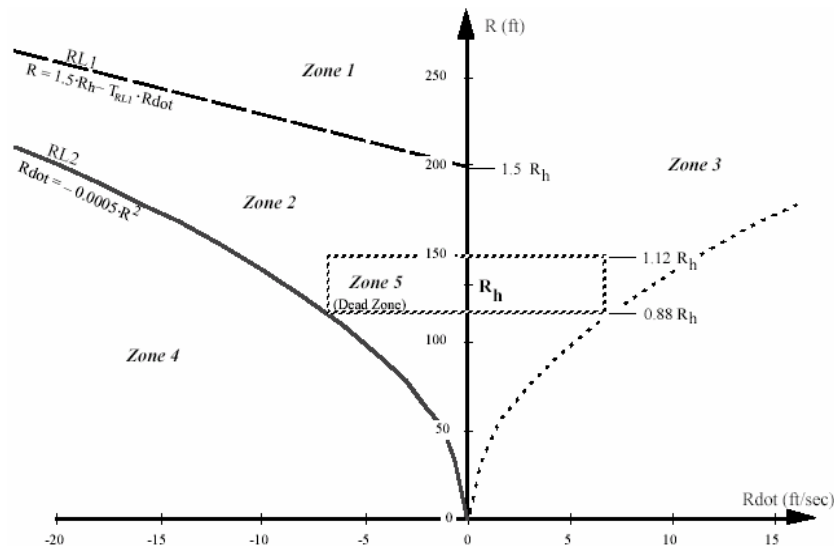
Figure 1.4 – Mappa regionale del modello di Fancher e Bareket
