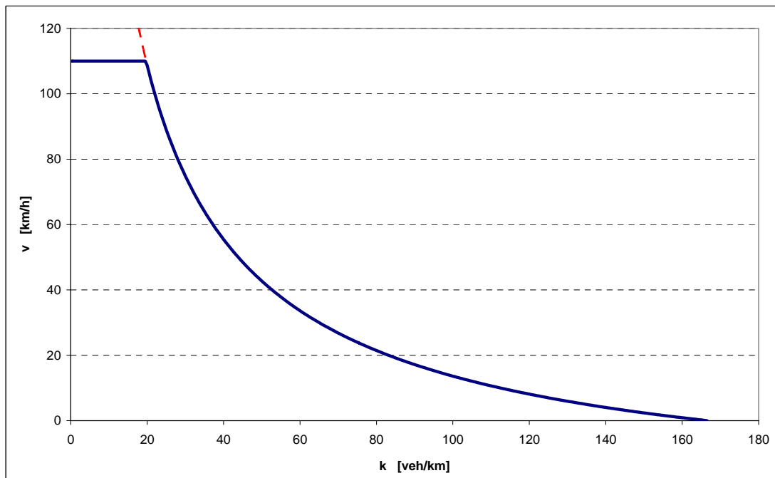
Figura 3.8 – Relazione velocità e densità per b < \hat{b} .
