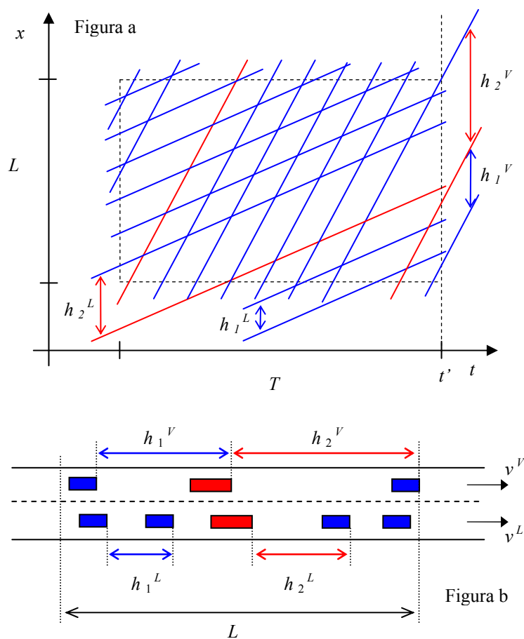
Figura 4.1 – Traiettorie dei veicoli nel diagramma spazio-tempo (a) e foto aerea nell'istante t' (b) per uno scenario di traffico stazionario a due corsie e due classi di veicoli.
