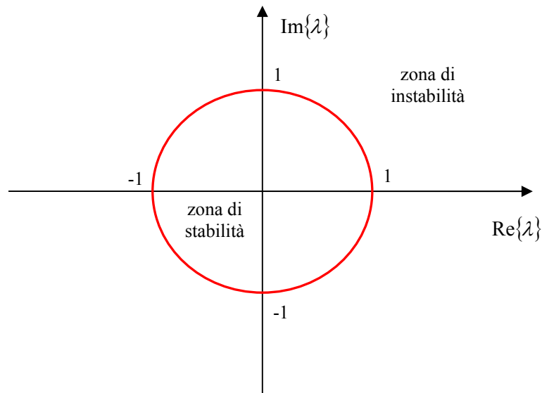
Figura 3.15 – Cerchio unitario per sistemi a tempo discreto.
