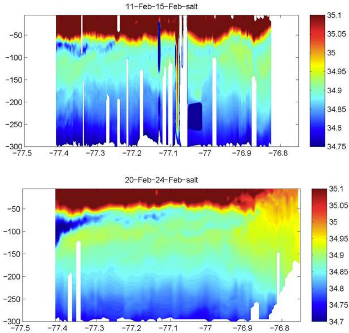
Abbildung 1: Salzgehaltsmessungen des Gleiters IFM12 vor Pisco. Um den gesamten Transekt zu vermessen, benötigt der Gleiter ca. 4 Tage. Die obere Grafik zeigt die übermittelten Messdaten vom 11. bis zum 15.02.2013, die untere Daten vom 20. bis zum 24.02.2013.
