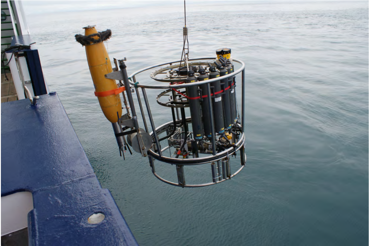
Abb.: Die profilierende Mikrostruktursonde BAKLAN (entwickelt am Shirshov Institut für Ozeanologie, Kaliningrad) wird mit der CTD zu Wasser gebracht.
