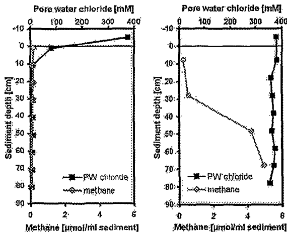
Abbildung 2: Typischer Konzentrations-Tiefen-Verlauf von Chlorid (schwarze Quadrate) und Methan (graue Kreise) an einer stark SGD-beeinflußten Lokation (links), bzw. einer unbeeinflußten Kontrollstation (rechts).
