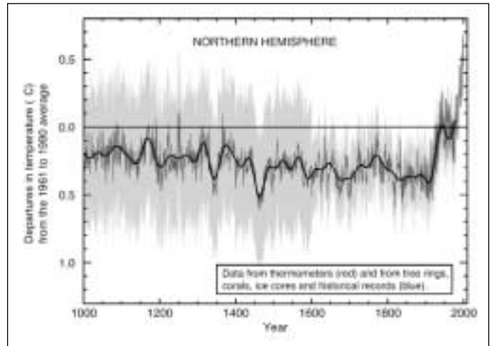
Abb. 2: Temperatur der Nordhalbkugel in den letzten 1000 Jahren (Quelle: IPCC 2001)
