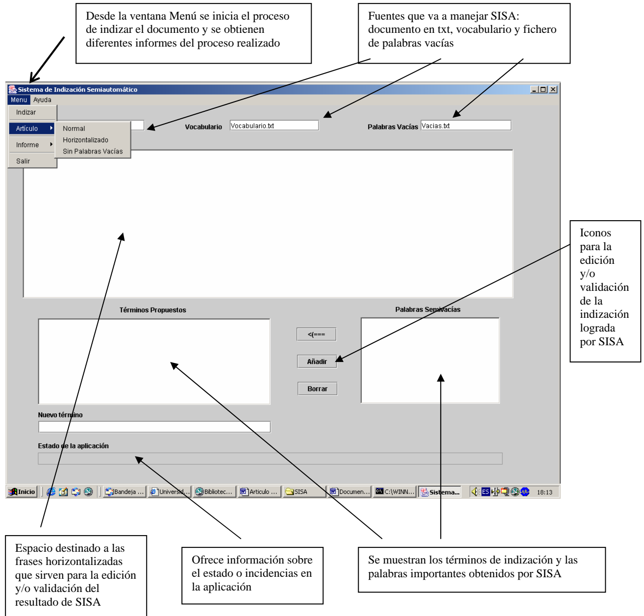
Figura 1: Explicación de la interfaz de SISA (v.1)
