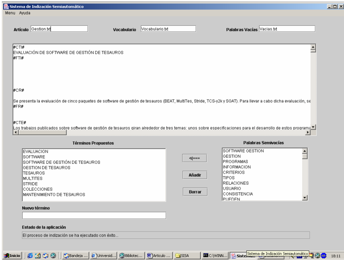
Figura 2: Pantalla de SISA una vez que ha indizado un documento:
