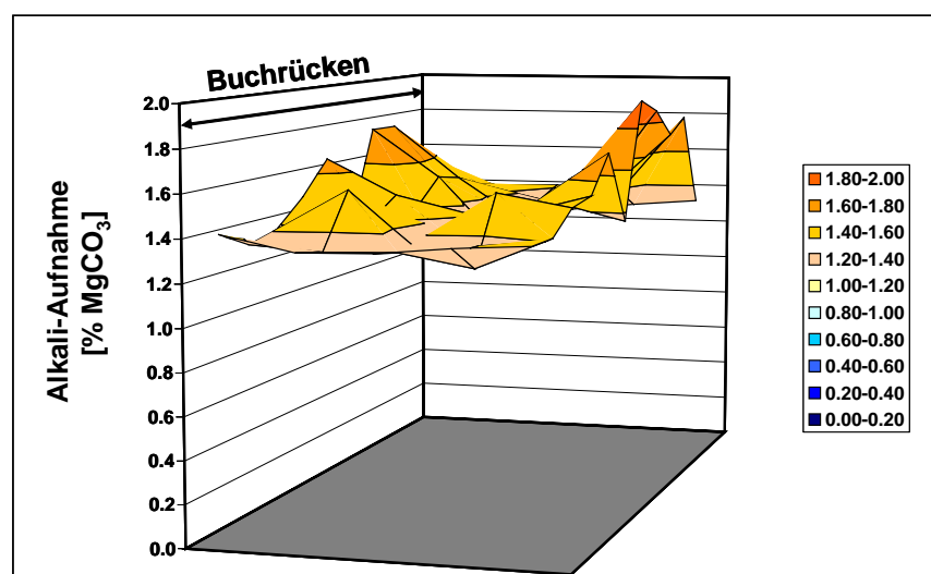
Abbildung 3: Homogenität der Behandlung über eine Buchseite. Die Alkaliaufnahme liegt zwischen 1.30 und 1.85% \text{MgCO}_3 – die Behandlung ist vollständig und recht homogen (bei anderen Massenentsäuerungsverfahren treten zwischen Buchmitte und Nähe Buchrücken Gradienten bis zu Faktor 10 auf).
