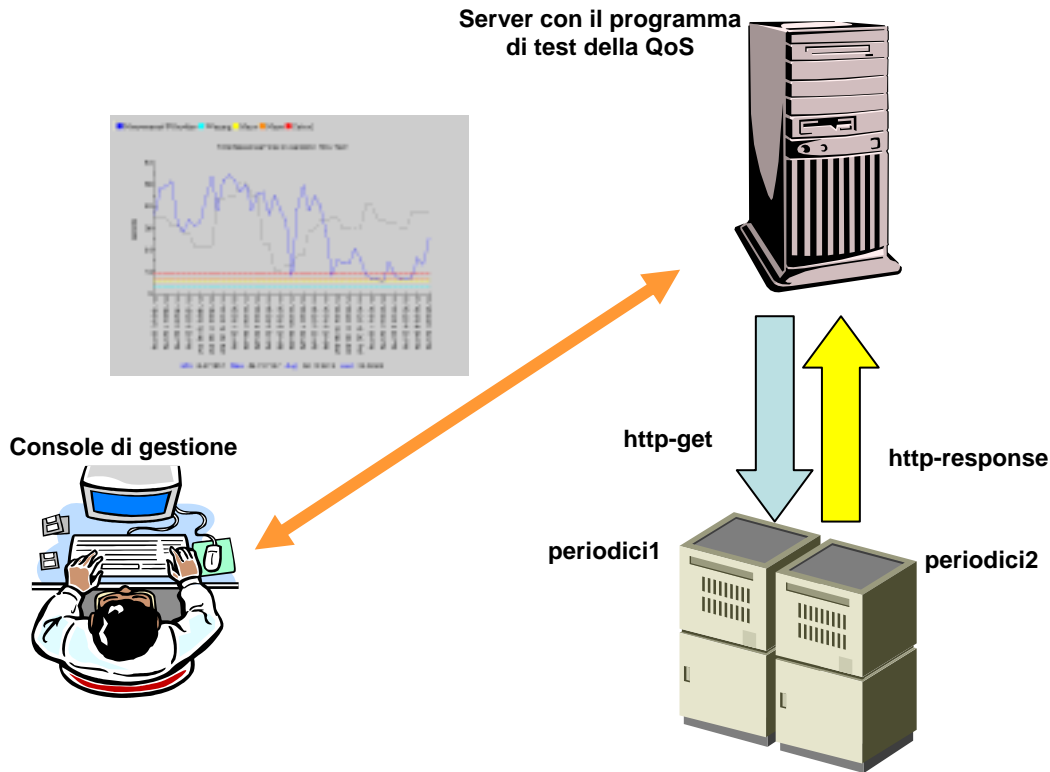
Fig.8 – Architettura utilizzata per i test di QoS dell’Emeroteca Virtuale
