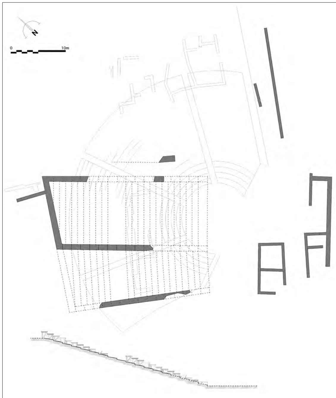
Fig. 4 – Efestia. Ipotesi di restituzione della fase lignea del teatro (punteggiato), in grigio le klimakes
