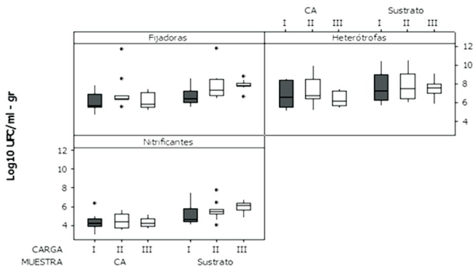
Figura 3. Distribución de Bacterias en el Humedal control. CA: Columna de Agua. En el eje x se muestran los niveles de la carga hidráulica (ch): I ( Q_d: 1.7 \text{ m}^3 \text{ d}^{-1} ); II ( Q_d: 2.6 \text{ m}^3 \text{ d}^{-1} ) y III ( Q_d: 3.5 \text{ m}^3 \text{ d}^{-1} ).
