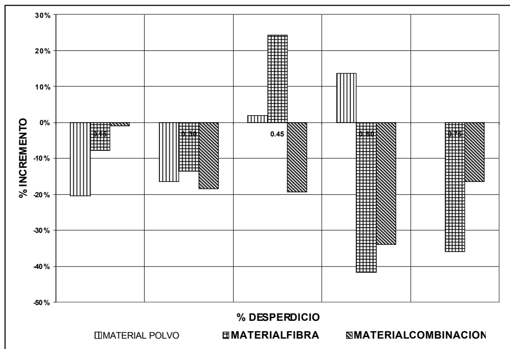
Figura 14. Efecto del desperdicio en el ahuellamiento
