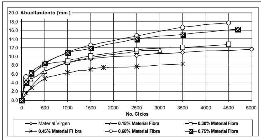
Figura 12. Variación del ahuellamiento con respecto al porcentaje de llanta usada en forma de tiras
