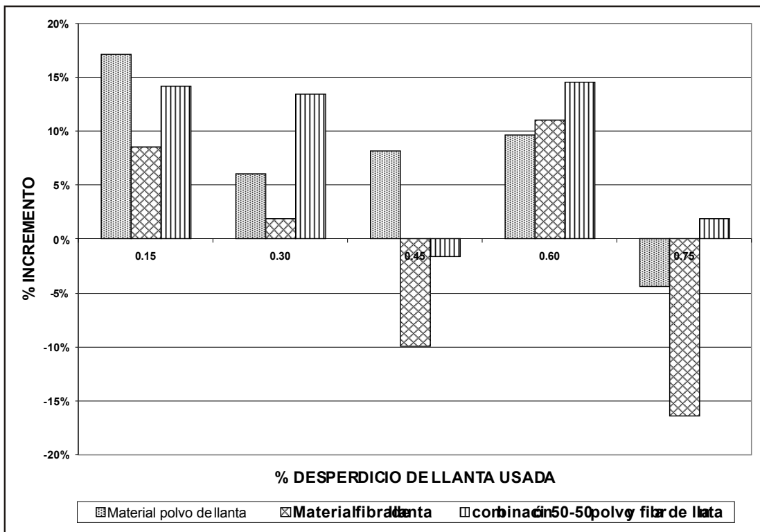
Figura 7. Incremento de la estabilidad con respecto a la adición de desperdicio de llanta usada para un nivel de energía de compactación de 50 golpes por cara
