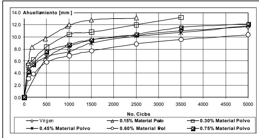
Figura 11. Variación del ahuellamiento con respecto al porcentaje de llanta usada en forma de polvo
