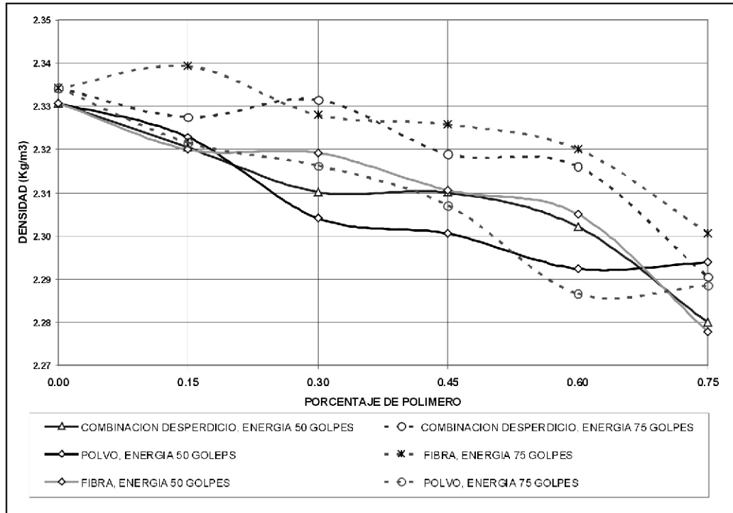
Figura 9. Variación de la densidad con respecto al porcentaje de desperdicio
