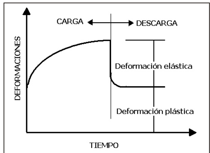
Figura 2. Comportamiento de materiales viscoelásticos
