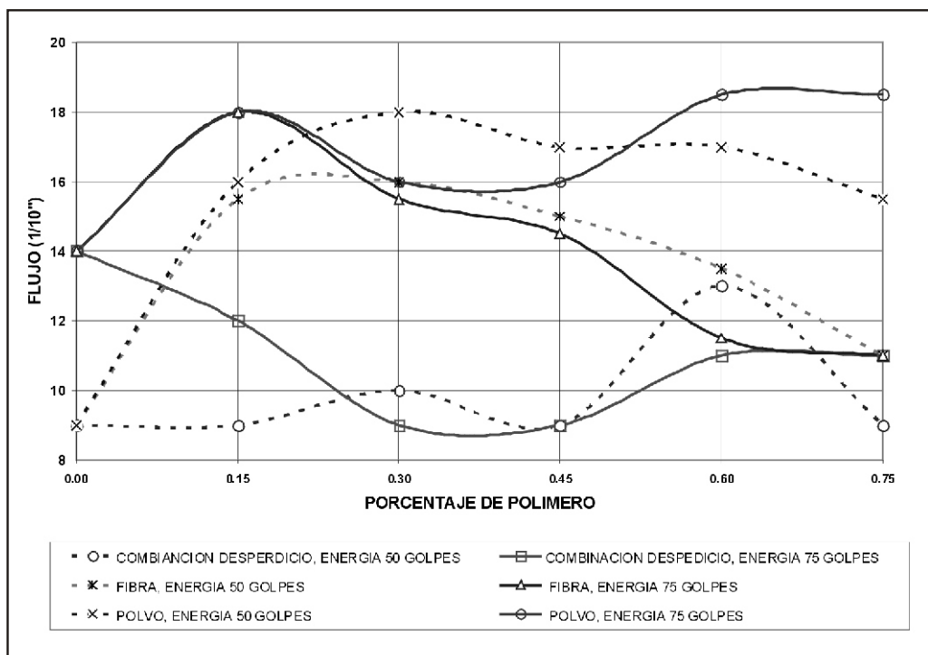
Figura 10. Variación del flujo con respecto al porcentaje de desperdicio
