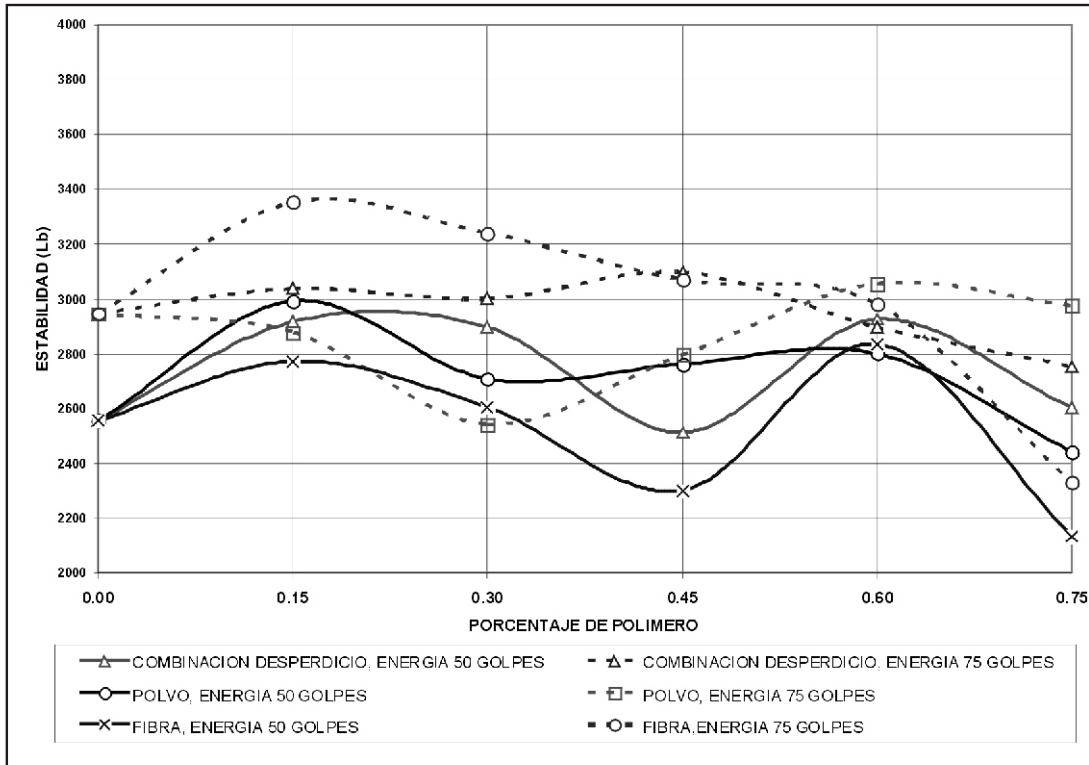
Figura 6. Variación de la estabilidad con respecto al porcentaje de desperdicio
