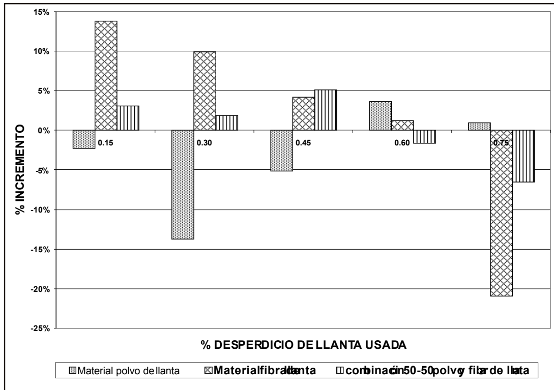
Figura 8. Incremento de la estabilidad con respecto a la adición de desperdicio de llanta usada para el nivel de energía de compactación de 75 golpes por cara
