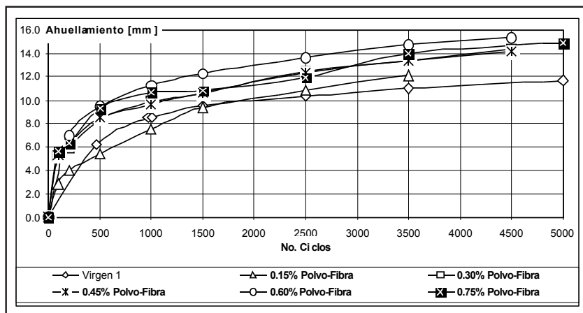
Figura 13. Variación del ahuellamiento con respecto al porcentaje de llanta usada con combinación de polvo y fibra
