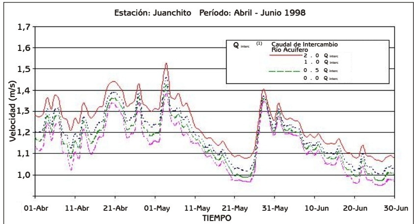
Figura No. 5 - Análisis de Sensibilidad del Modelo Hidrodinámico - Influencia del Intercambio Río - Acuífero en la Velocidad
