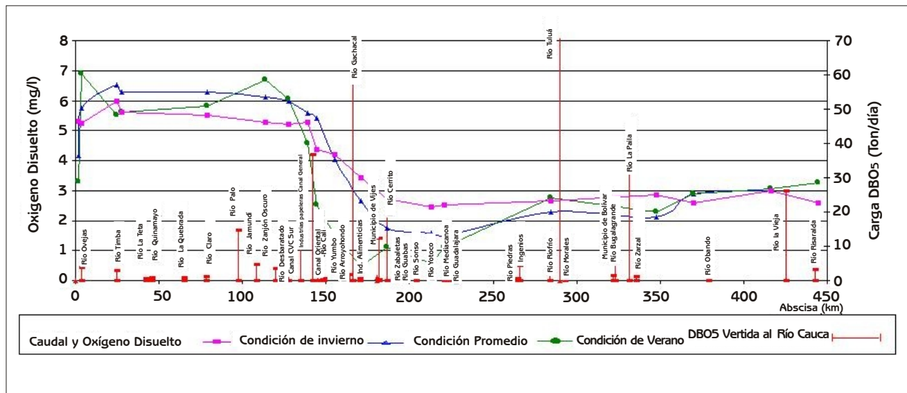
Figura No. 3 - Variación del Oxígeno Disuelto en el Tramo Salvajina - La Virginia
