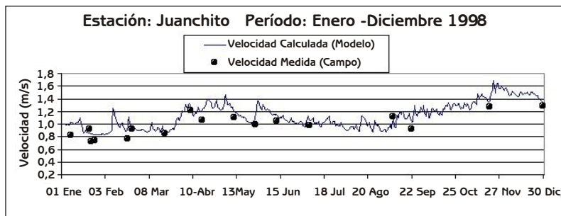
Figura No. 4 - Calibración Modelo Hidrodinámico Velocidad Calculada Vs. Velocidad Medida
