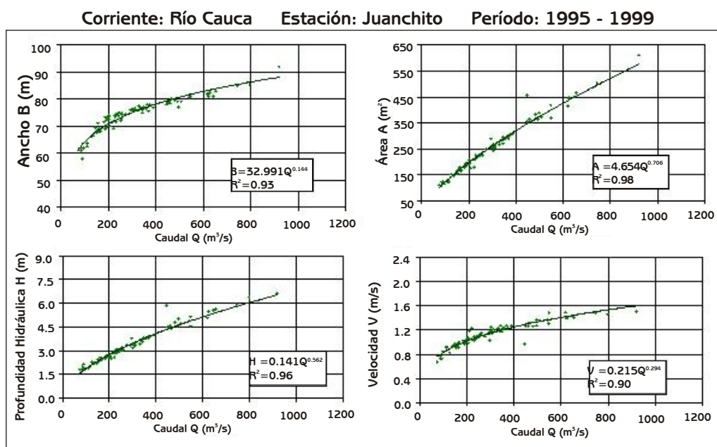
Figura No. 1 - Relaciones Caudal vs. Parámetros Hidráulicos y Geométricos
