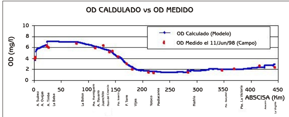
Figura No. 6 Calibración del Modelo de Calidad del Agua
