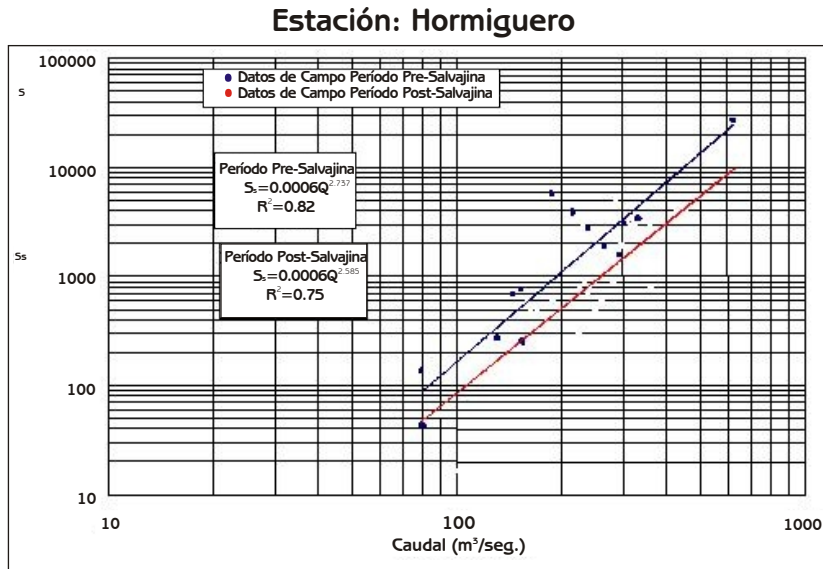
Figura No. 2 - Caudal vs. Carga Total en Suspensión del Río Cauca
