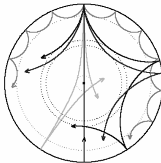
2. ábra. A különböző rezgések a csillag különböző mélységéig terjednek. Két közeli frekvencia közel azonos mélységig terjed. A frekvenciák mért különbsége a két fordulópont közötti réteg fizikai paramétereit adja. A Nap rezgései csak a külső rétegben terjednek. Más csillagokban a mélyebb rétegeket is vizsgálni lehet.
