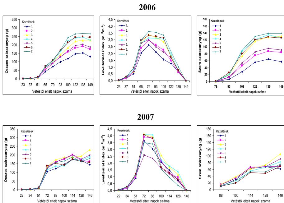
8. ábra. Az istállótrágya és a műtrágya hatása az összes szárazanyag termelés, a levélterület index (LAI) és a szemtermés időbeni növekedésének dinamikájára két eltérő évjárathatásban
