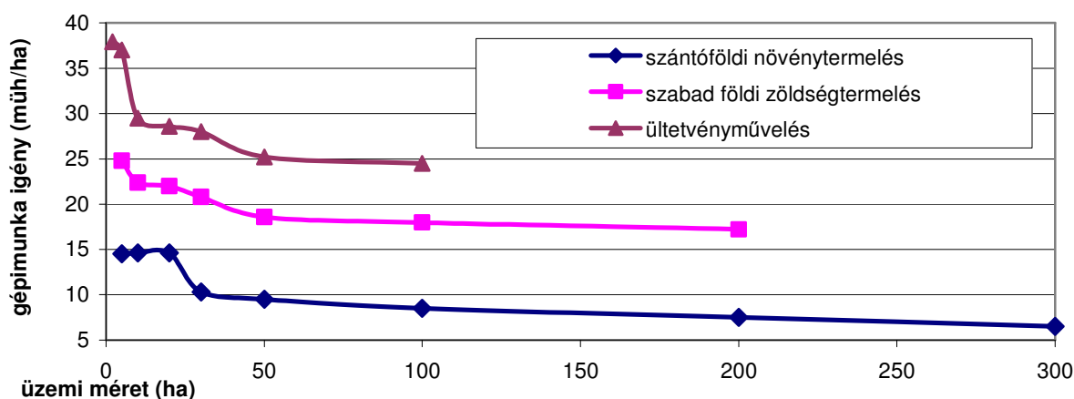
9. ábra: A hektáronkénti éves gépmunka igény az üzemi méret függvényében a különböző ágazatokban
