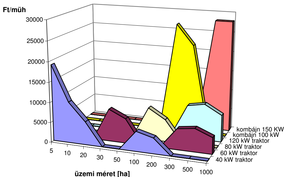
14. ábra: Az erőgép-kategóriák műszakóránkénti legalacsonyabb kalkulált fajlagos használati költsége a vizsgált üzemi méreteknél szántóföldi növénytermelés esetén
