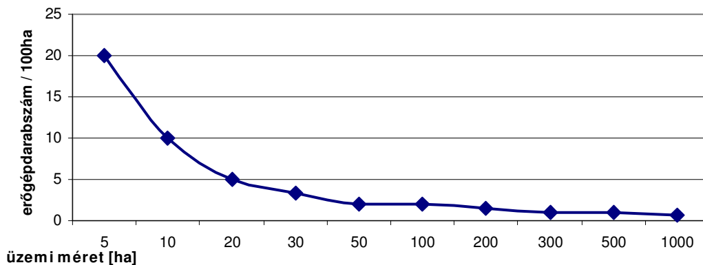
2. ábra: A 100 hektárra jutó fajlagos erőgépdarabszám a vizsgált üzemi méreteknél szántóföldi növénytermelés esetén
