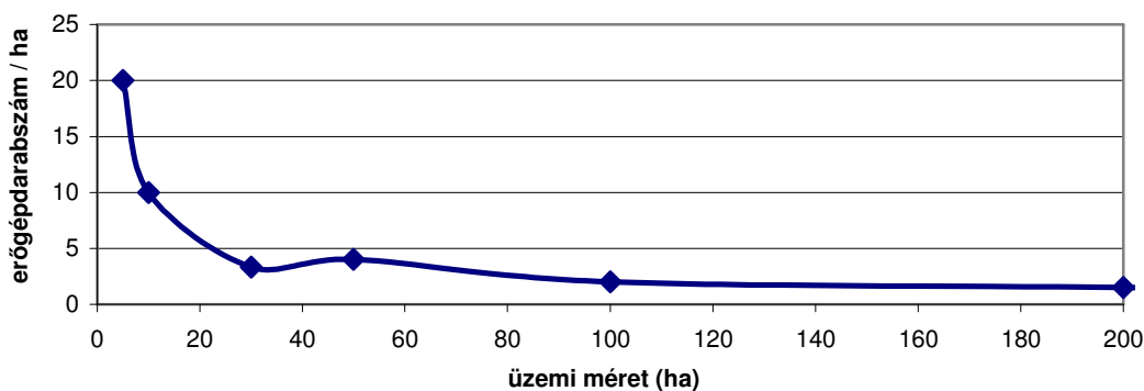
4. ábra: A 100 hektárra jutó fajlagos erőgépdarabszám a vizsgált üzemi méreteknél szabad földi zöldségtermelés esetén
