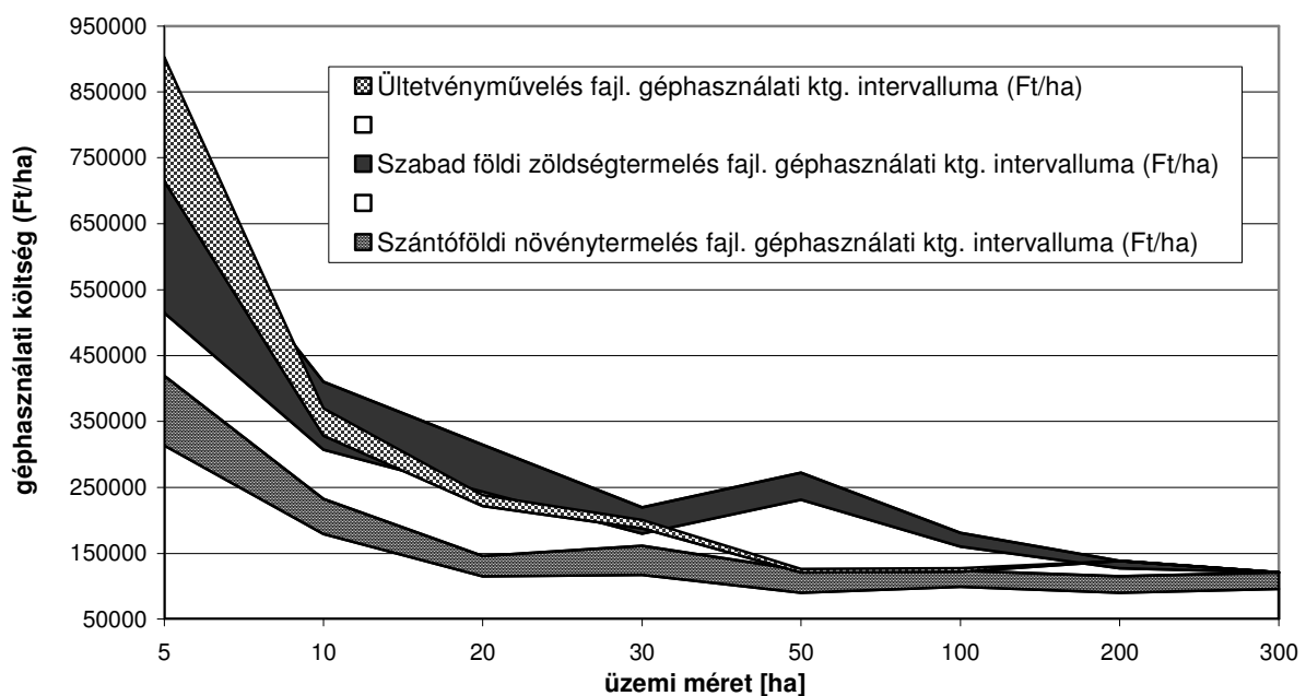
10. ábra: A fajlagos géphasználati költségek értéksávja a különböző ágazatoknál az üzemi méret függvényében
