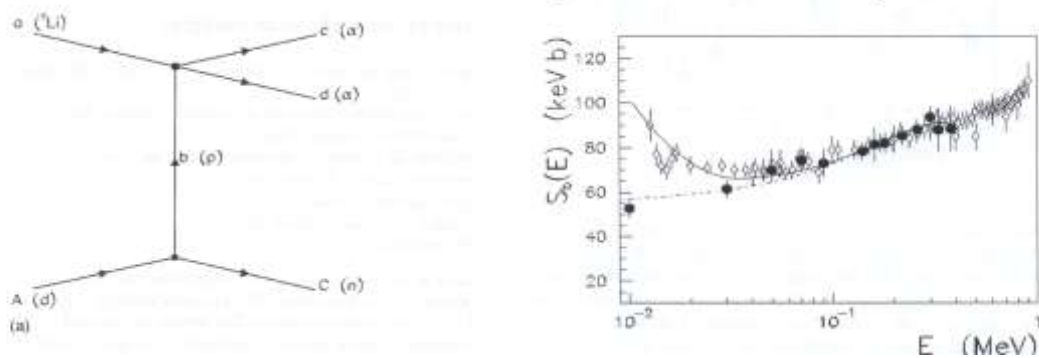
3. ábra. A THM módszer gráfja (balra) és a THM eredmények (vastag pontok) összehasonlítása a ^7\text{Li}(p,\alpha)^4\text{He} reakció (elektronárnyékolással bíró) direkt mérésével (jobbra).
