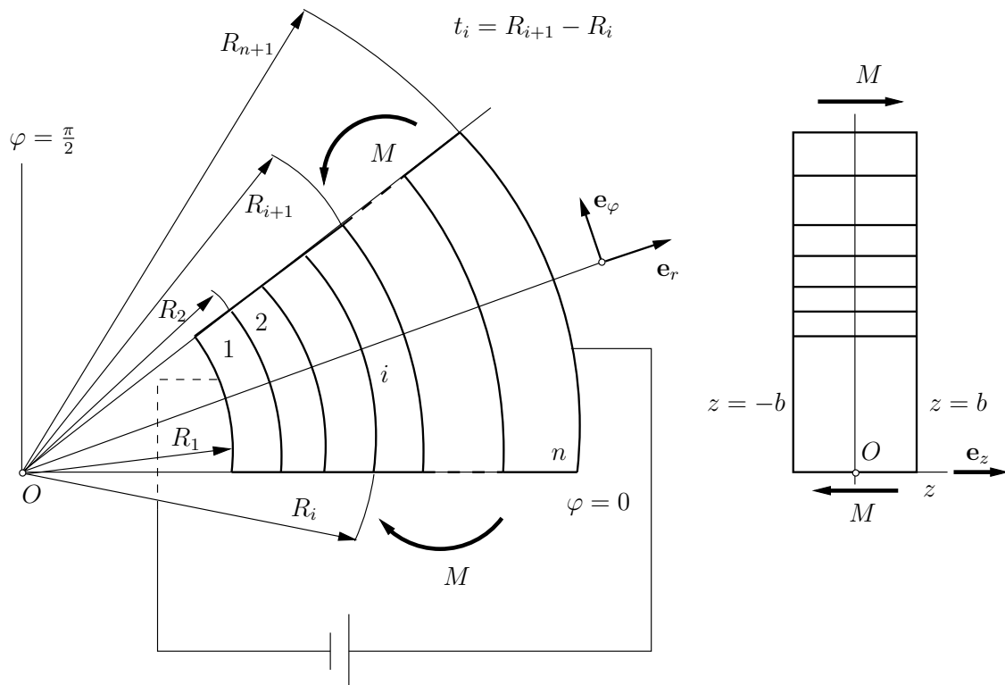
14. ábra. Állandó görbületű, rétegzett piezoelektromos rúd.
