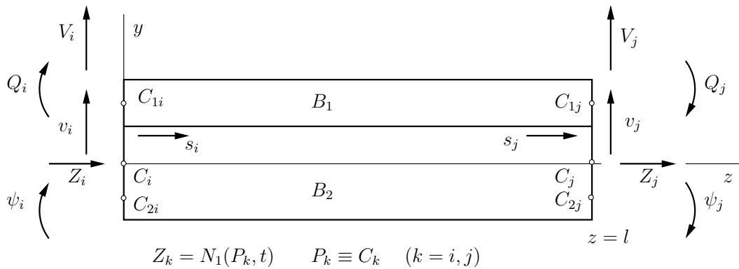
10. ábra. Kétcsomópontú rétegzett, részlegesen kapcsolt rúdelem.
