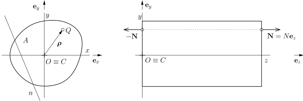
2. ábra. Excentrikusan húzott z -homogén rúd.
