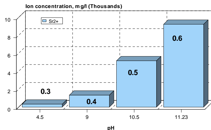
3. ábra: A pH hatása a SrSO 4 oldhatóságára ( C_{\text{DTPA}}=0,1 \text{ mol/l} )
