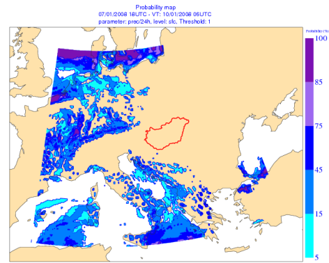
6. ábra: (a) Bélyeg diagram mind a 11 ensemble tagra. Az ábrázolt paraméter a 24 órás csapadékösszeg. Az előrejelzés kiinduló időpontja 2008. január 7., 18 UTC. Az előrejelzés érvényességi ideje 2008. január 9., 06 UTC - 2008. január 10., 06 UTC. (b) Valószínűségi térkép. Az ábrázolt paraméter: a 24 órás csapadékösszeg mennyisége nagyobb, mint 1 mm. Az előrejelzés kiinduló időpontja 2008. január 7., 18 UTC. Az előrejelzés érvényességi ideje 2008. január 9., 06 UTC - 2008. január 10., 06 UTC.
