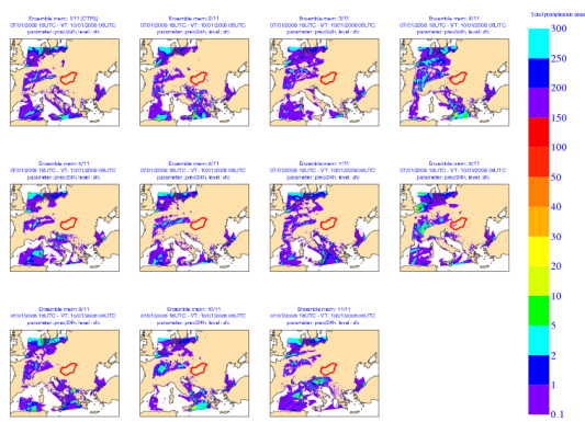
6. ábra: (a) Bélyeg diagram mind a 11 ensemble tagra. Az ábrázolt paraméter a 24 órás csapadékösszeg. Az előrejelzés kiinduló időpontja 2008. január 7., 18 UTC. Az előrejelzés érvényességi ideje 2008. január 9., 06 UTC - 2008. január 10., 06 UTC. (b) Valószínűségi térkép. Az ábrázolt paraméter: a 24 órás csapadékösszeg mennyisége nagyobb, mint 1 mm. Az előrejelzés kiinduló időpontja 2008. január 7., 18 UTC. Az előrejelzés érvényességi ideje 2008. január 9., 06 UTC - 2008. január 10., 06 UTC.
