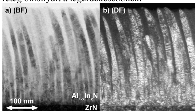
2. ábra: Az \text{AlInN} nanofű keresztmetszete világos ill. sötét látóterű képen.
